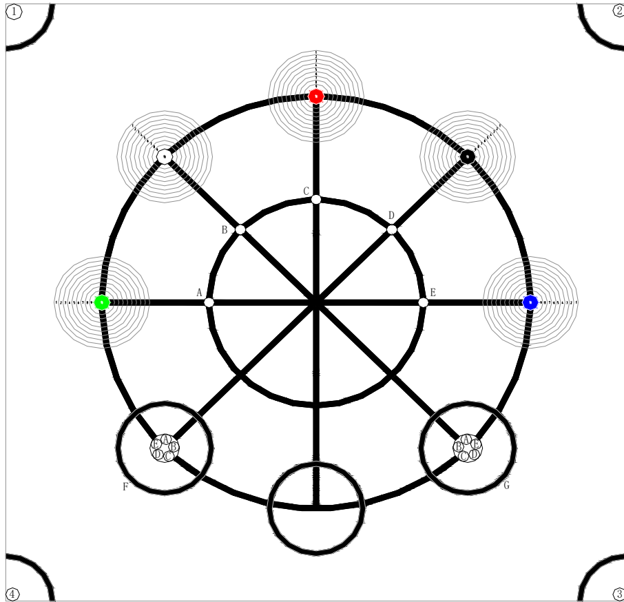
图 1 比赛场地示意图
